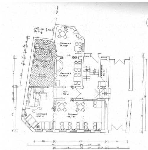
Grundriss EG
