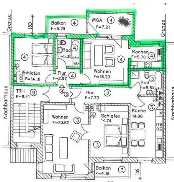
Grundriss
